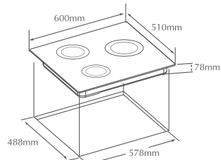
HOB EEG60301
