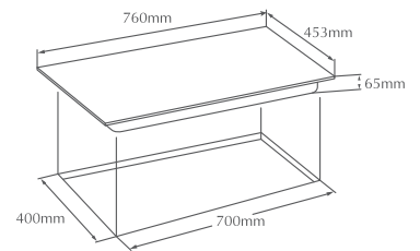
HOB EIG76203
