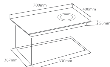
HOB MEG70201
