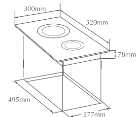
HOB EEG30202
