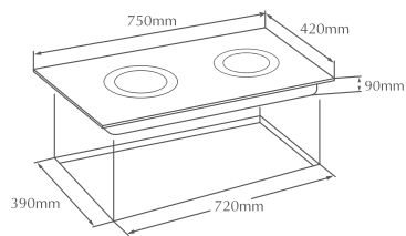
HOB EEG75201
