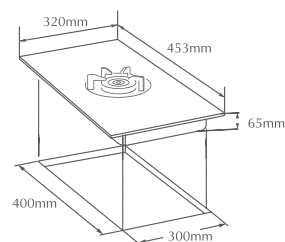
HOB GEG30103
