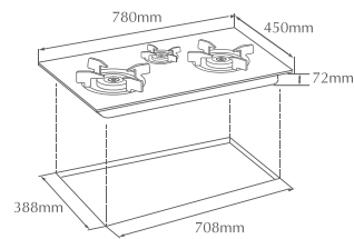
HOB GHG78312
